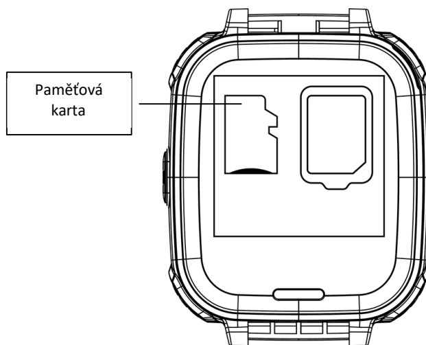
Obrázek 5 – Instalace paměťové karty
